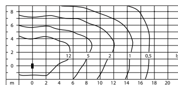
Diffusion lumineuse LED 14 W.
