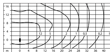
Diffusion lumineuse LED 176 W.
