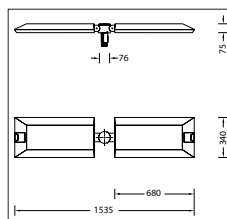
Diffusion lumineuse LED 218 W.
