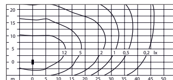
Diffusion lumineuse LED 218 W.
